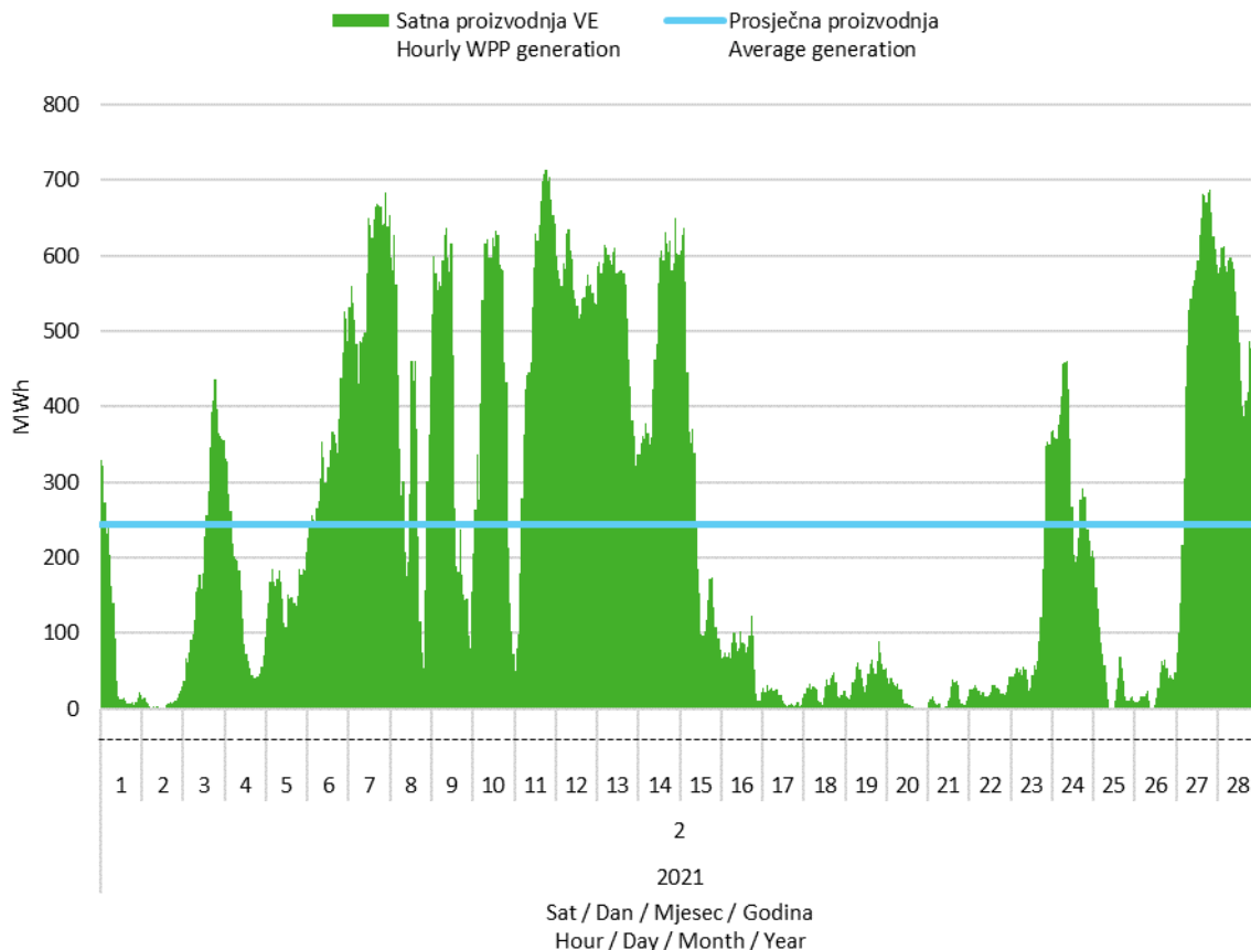
Slika 2 Satna proizvodnja svih vjetroelektrana u veljači 2021. godine Figure 2 Hourly generation of all wind power plants in February 2021
