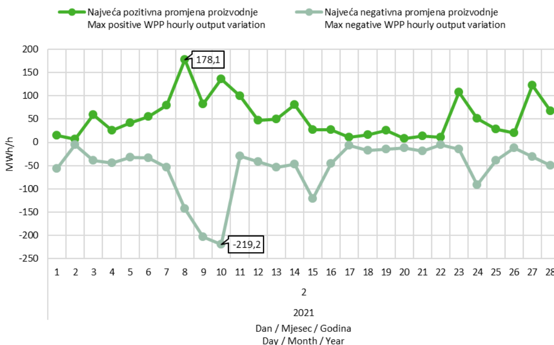
Slika 9 Maksimalna pozitivna i maksimalna negativna promjena satne proizvodnje VE u veljači 2021. godine
