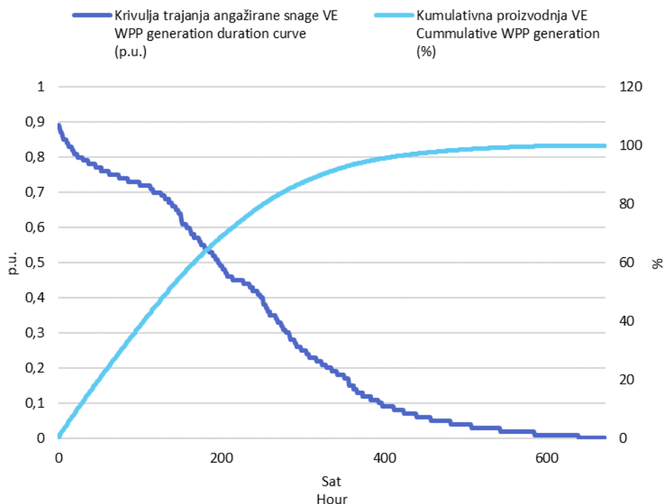
Slika 3 Krivulja trajanja angažirane snage svih VE i kumulativna proizvodnja VE u veljači 2021. godine u jediničnim vrijednostima
