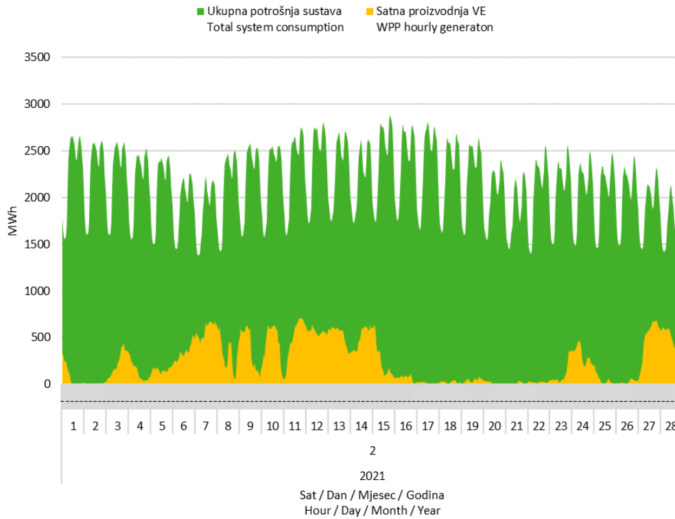
Slika 7 Usporedba satnog dijagrama opterećenja sustava i proizvodnje vjetroelektrana u veljači 2021. godine
