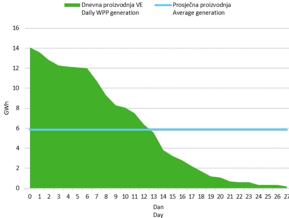
Slika 6 Krivulja trajanja dnevne proizvodnje vjetroelektrana u veljači 2021. godine
