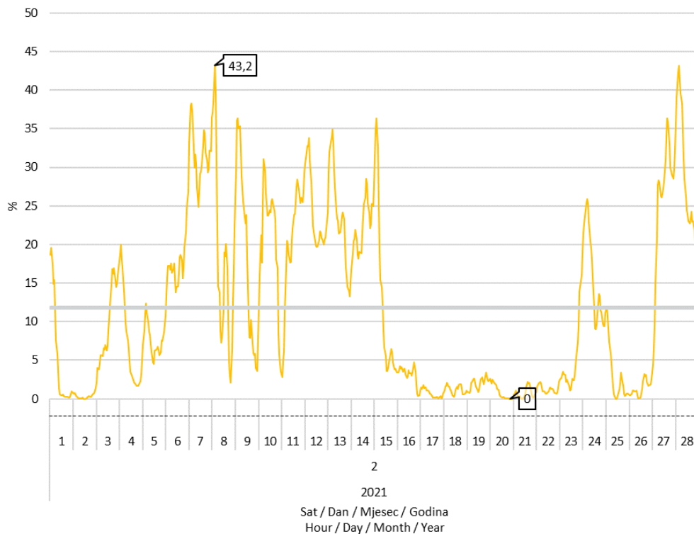
Slika 8 Udio proizvodnje vjetroelektrana u pokrivanju satnog opterećenja elektroenergetskog sustava u veljači 2021. godine
