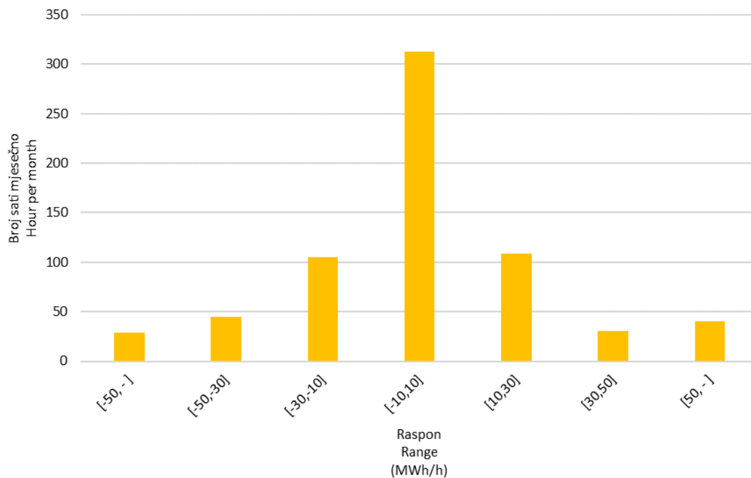
Slika 10 Statistička raspodjela satnih promjena proizvodnje VE u veljači 2021. godine Figure 10 Statistical distribution of WPP hourly output variations in February 2021
