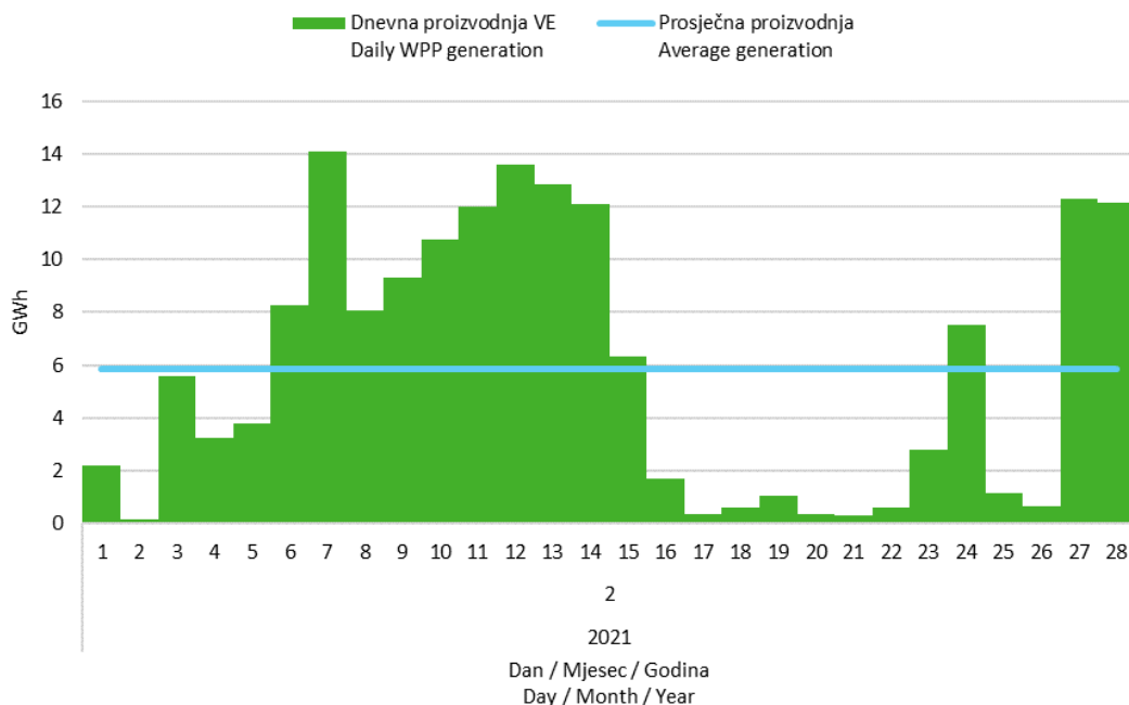
Slika 5 Dnevna proizvodnja svih vjetroelektrana u veljači 2021. godine Figure 5 Daily generation of all wind power plants in February 2021
